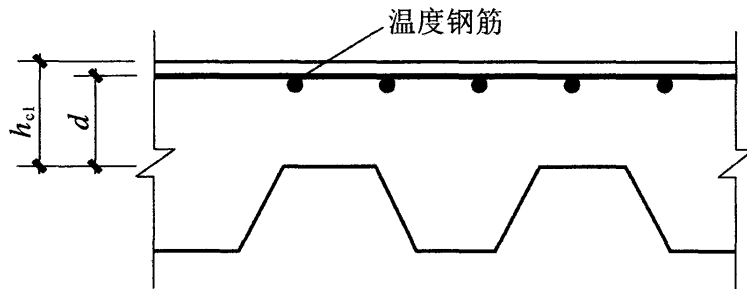
图 D.0.4 组合楼板的几何参数
