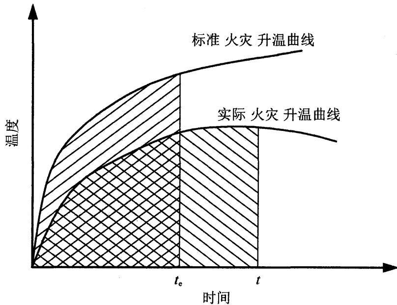
图 9 等效曝火时间 t_e
