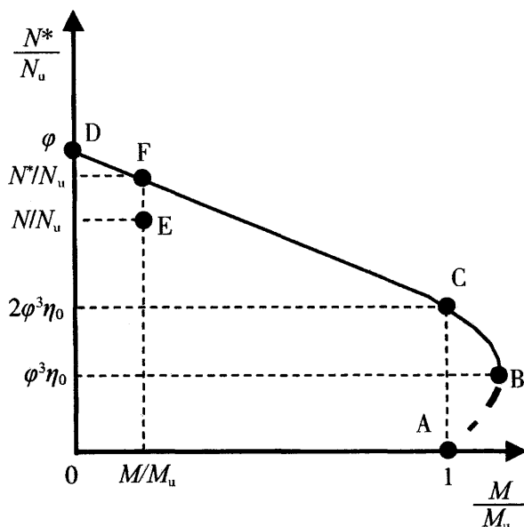
图 13 N^*/N_u-M/M_u 关系
