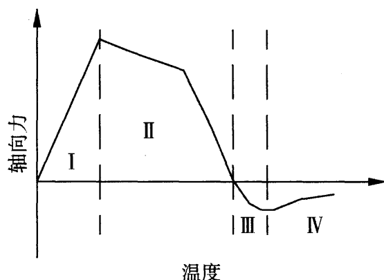
图 11 两端约束钢梁轴力随温度的变化图
