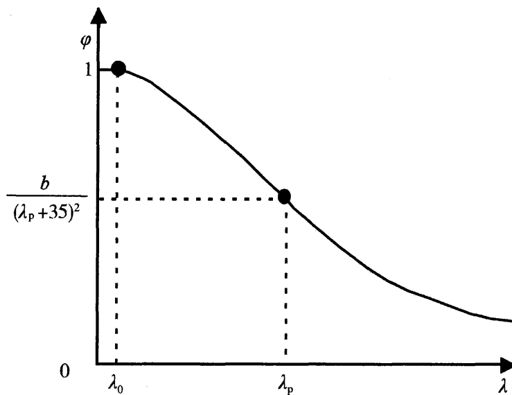
图 14 \varphi-\lambda 关系曲线示意图
