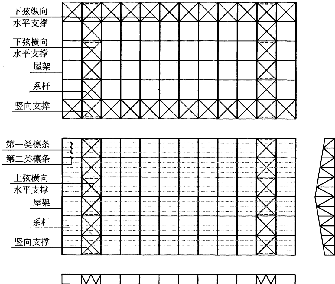
图 1 典型的屋盖结构体系
