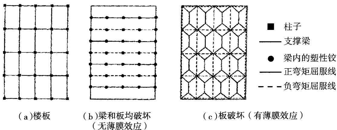
图 18 楼板弯曲破坏的形式
