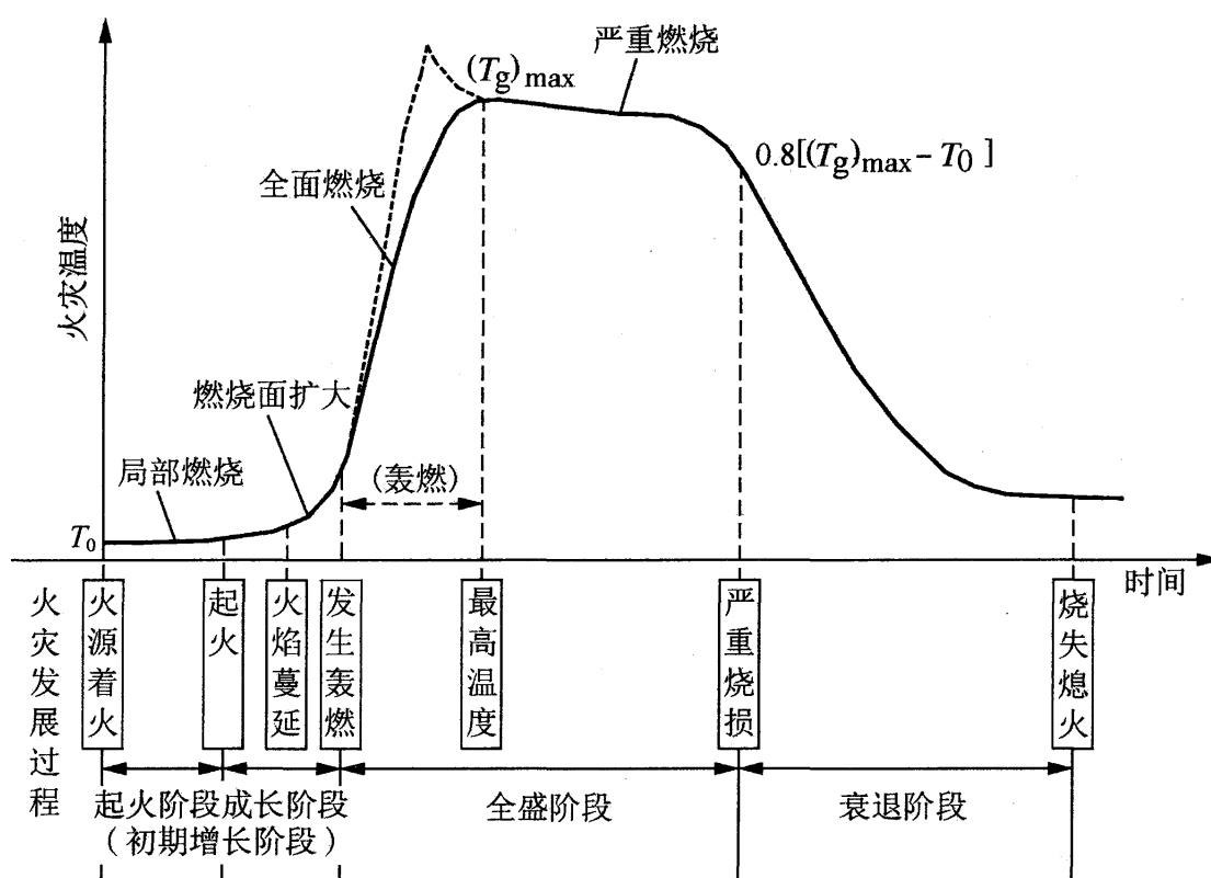
图7 一般室内火灾的发展过程
